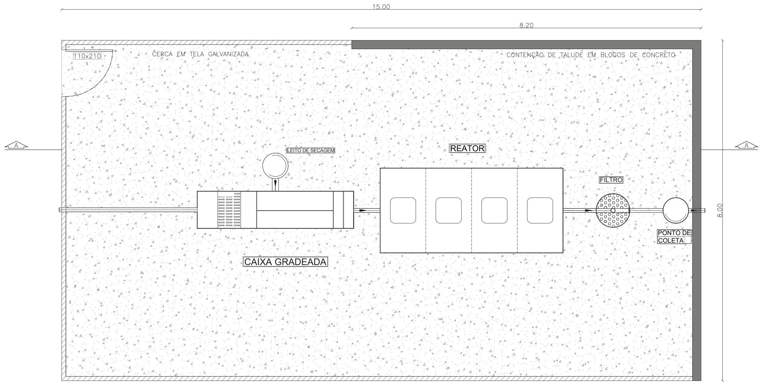
PLANTA BAIXA esc 1:50
