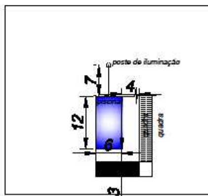
LOCAÇÃO PARA ESCORREGADOR BALEIA
